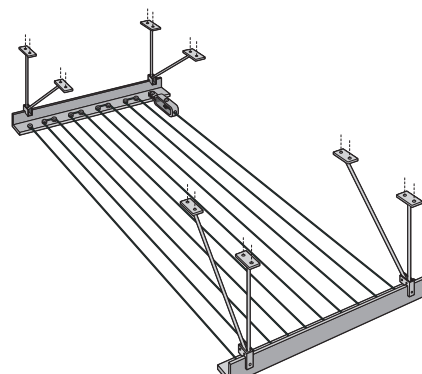
Decke-Decke-Montage DD
